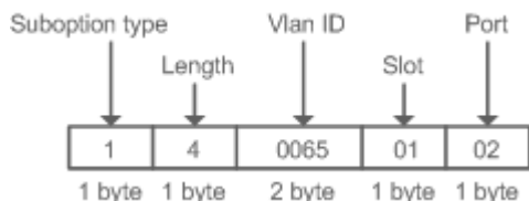
图 3-8 Agent Remote ID
