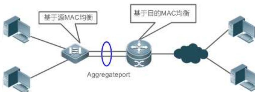
图 3-1 AP 链路聚合及流量平衡示意图
