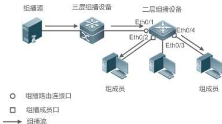
图 1-6 IGMP Snooping 的两类端口
