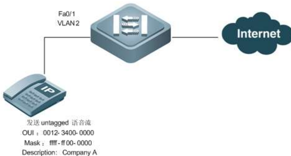
图 5-2 Voice VLAN 手动模式配置组网图
