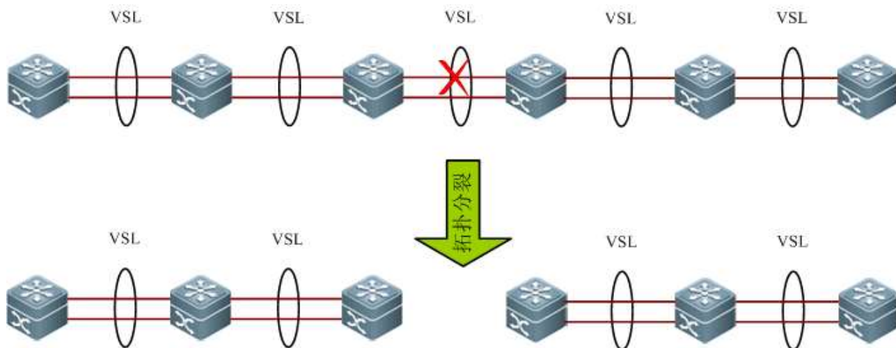
图 7-31 拓扑分裂
