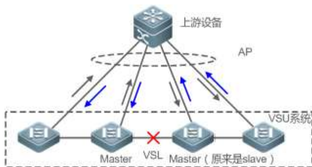
图 7-14 聚合口的上下游方式多主机检测
