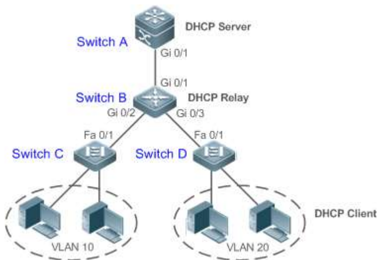
图 3-3DHCP Relay 组网拓扑图
