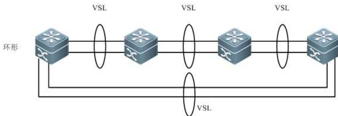
图 7-9 环形拓扑
