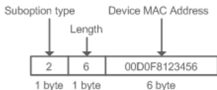
图 3-8 Agent Remote ID
