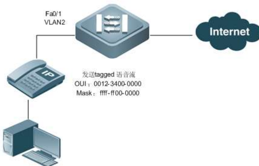
图 5-1 Voice VLAN 自动模式配置组网图
