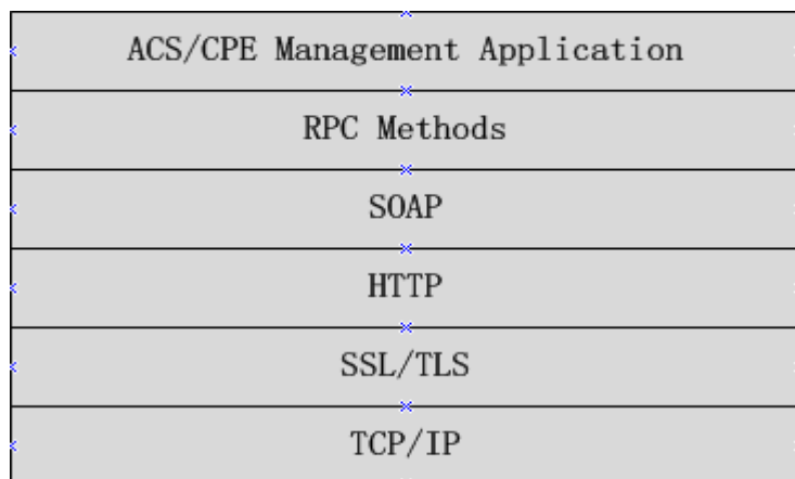
图 6-2 CWMP 的协议结构
