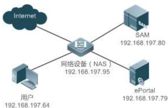
图 4-1 Web 认证方案网络拓扑图
