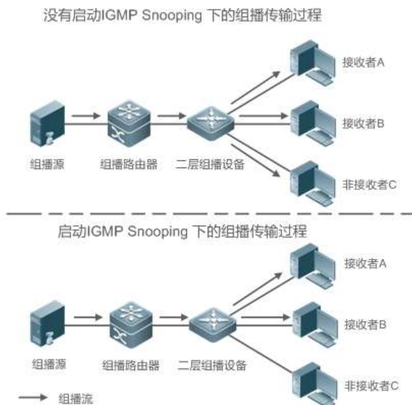
图 1-1 IP 组播流在 VLAN 内的转发 (二层组播设备启动 IGMP Snooping 前后的对比)
