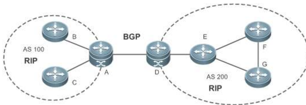
图 3-2 RIP 与 BGP 互联
