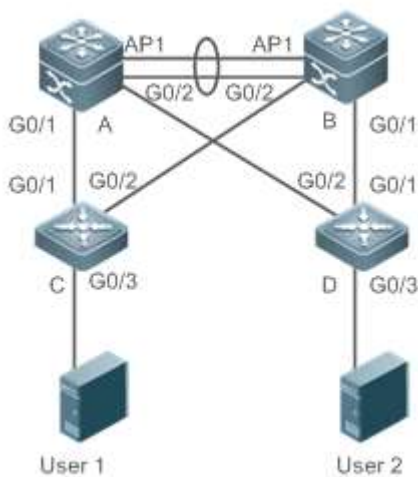
图 6-1 MSTP+VRRP 双核心拓扑
