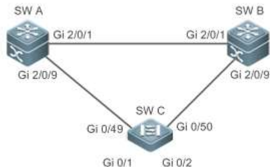
图 2-4 中链路出现单向或者双向故障进而导致 STP 协议失效，汇聚设备与汇聚设备之间以及汇聚与接入设备之间启用 RLDP 单向和双向检测，为了防止汇聚设备下联被错误的接入而出现环路，汇聚设备与接入设备的下联端口均开启 RLDP 环路检测；为了防止接入设备下联被错误的接入而出现环路，接入设备的下联端口均开启 RLDP 环路检测
