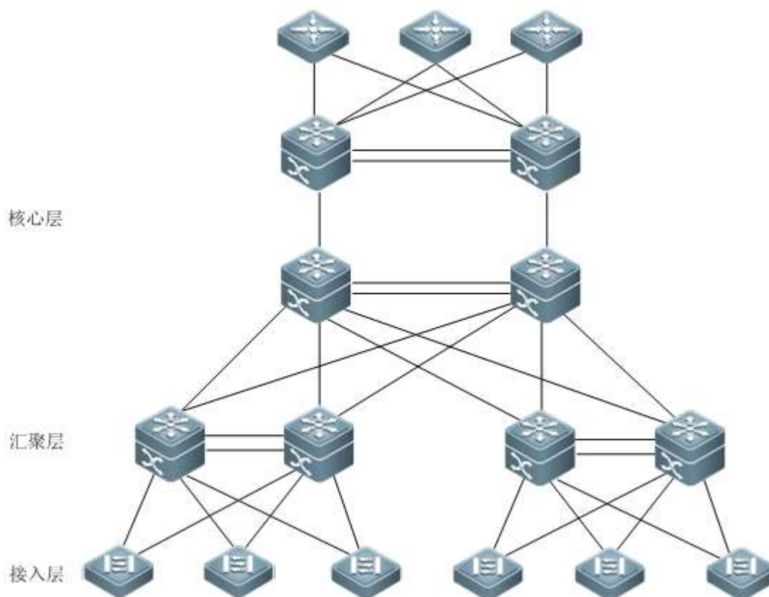
图 7-1 传统网络结构
