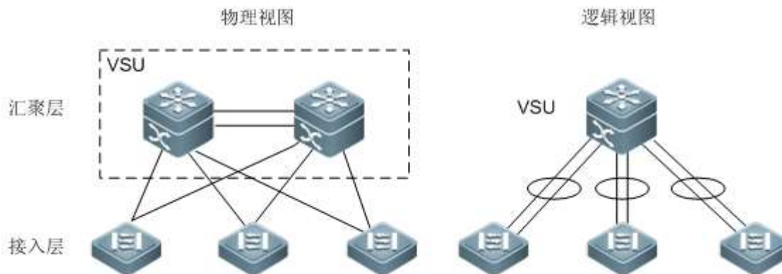
图 7-5 汇聚层的 VSU
