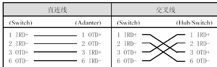
图A-3 100BASE-TX/10BASE-T双绞线联接方式
