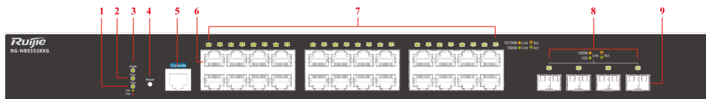
图1-6 RG-NBS5528XG 前面板示意图
