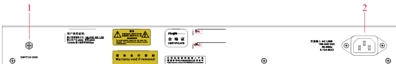
图1-7 RG-NBS5528XG 后面板示意图
