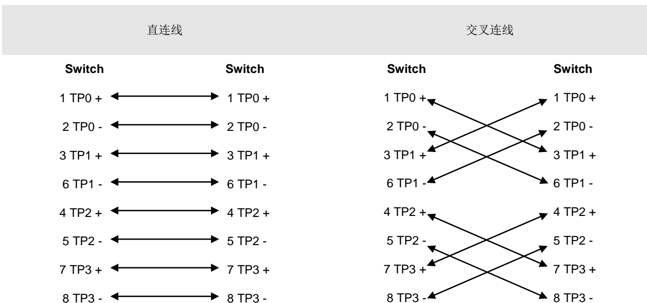
图 A-1 1000BASE-T 四对双绞线示意图
