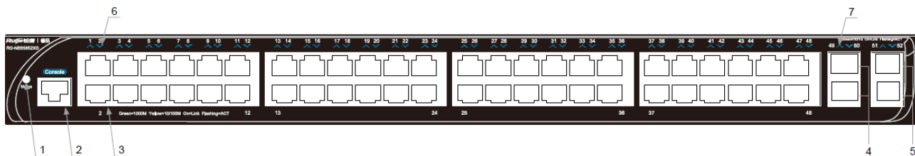
图 1-5 RG-NBS5652XG 前面板示意图
