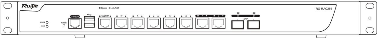
图 1-2 RG-RAC256 无线控制器产品后面板
